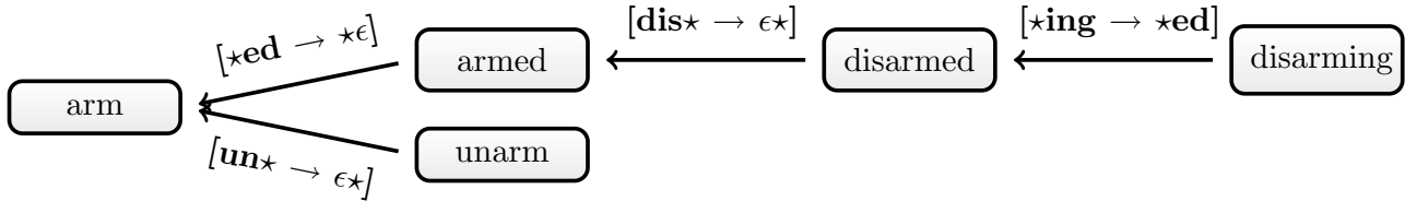
FIG. 2 – ADM des mots anglais dérivés de arm .
