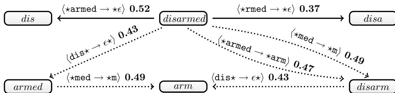
FIG. 3 – Graphe des mots atteignables depuis le mot anglais disarmed . Les arcs en pointillés sont ceux considérés lors du calcul du score entre disarmed et arm .
