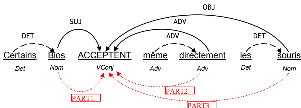
Figure 20 Schéma de combinaison les flèches au-dessus des mots correspondent aux liens donnés par Syntex. Nous indiquons en pointillé les liens qui ne seront pas considérés. Les flèches sous les mots correspondent aux participants annotés manuellement.
