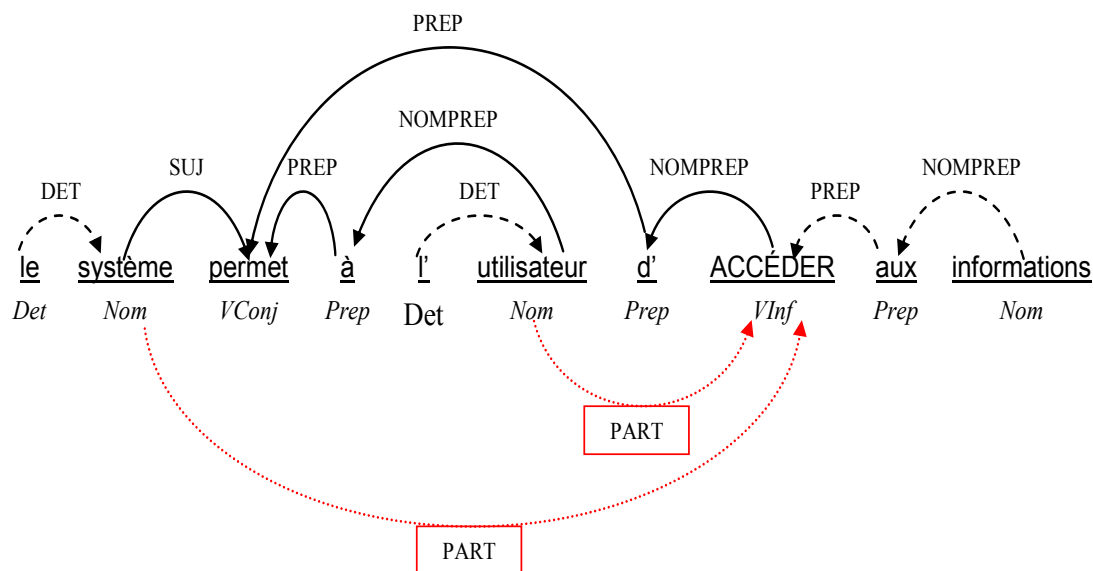
Figure 70 Dépendance Lexie| permettre à ... de ... (Règle 28)( Règle 24)
