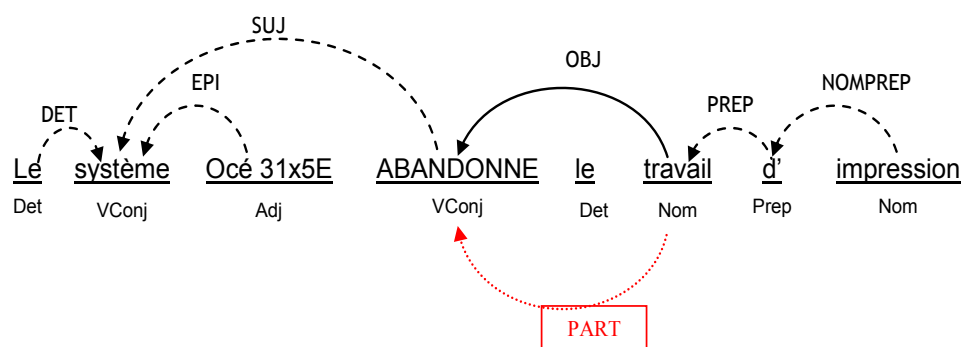
Figure 44 Dépendance Objet (OBJ) (Règle 3)
