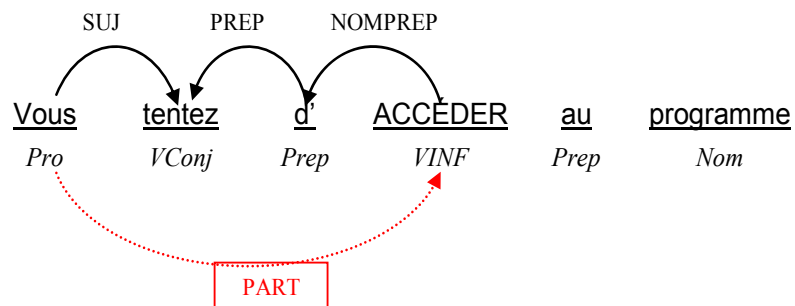
Figure 63 Dépendance Lexie| tenter de (Règle 19)
