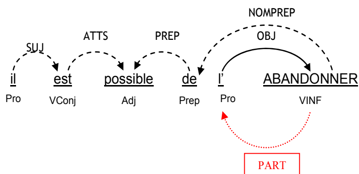
Figure 45 Dépendance Objet d'un pronom sujet (Règle 3)
