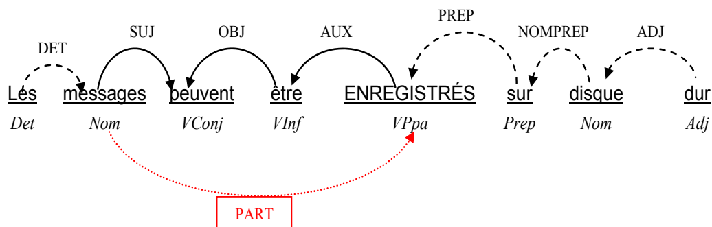
Figure 62 Dépendance Lexie|pouvoir+auxiliaire (Règle 18)
