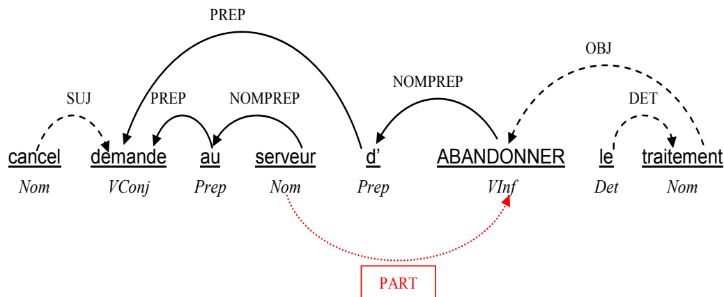
Figure 69 Dépendance Lexie| demander de (Règle 23)
